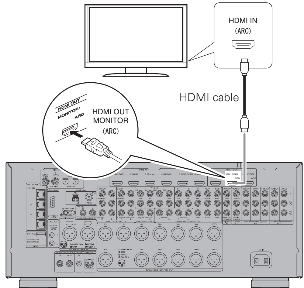
AV Pre Tuner (Rear panel)
