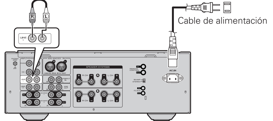
Amplificador (Panel trasero)
