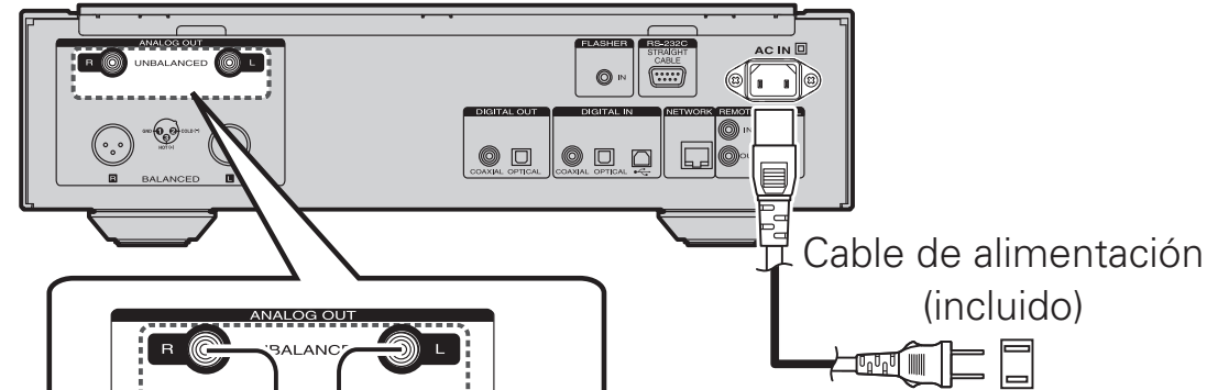
NA-11S1 (Panel trasero)
